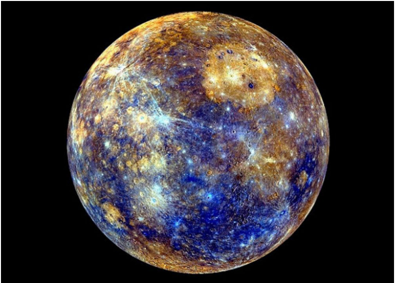
Меркурий — ближайшая к Солнцу планета
