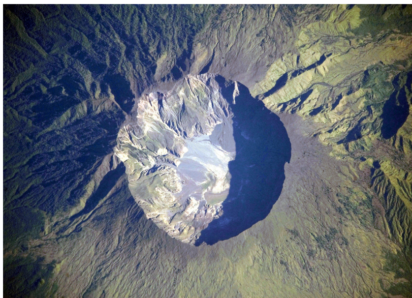
Кальдера вулкана Тамбора
